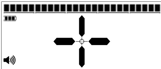
Stärkstes Objektsignal: Alle Diskriminierungsabschnitte sind eingeschaltet. Das Objekt befindet sich direkt unter der Mittellinie der Spule.
